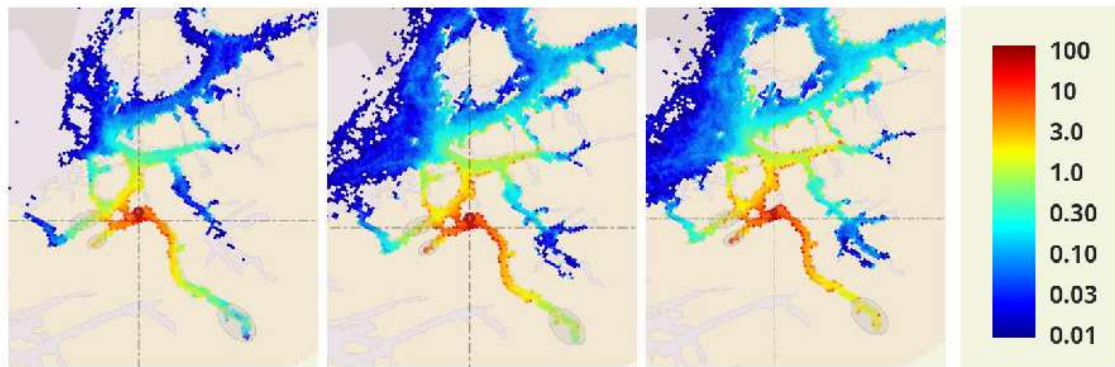
Figur 6: Strømsimulering lokalitet Ranem i ROMS-modell Nor Kyst 800 – 10, 20 og 30 dagers drift
