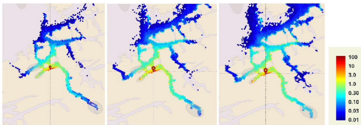
Figur 5: Strømsimulering lokalitet Slettnes i ROMS-modell Nor Kyst 800 – 10, 20 og 30 dagers drift
